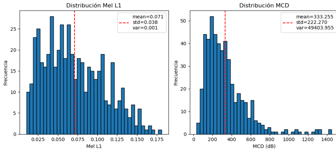
Figura 5.2: Gráficas que muestran los resultados de evaluar el conjunto de tests sobre el modelo P1 con las métricas Mel L1 y MCD.
