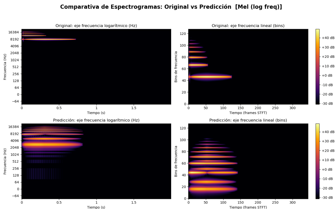
Figura 5.23: Espectrograma resultado de la predicción del audio de Benchmark: muy_agudo .
